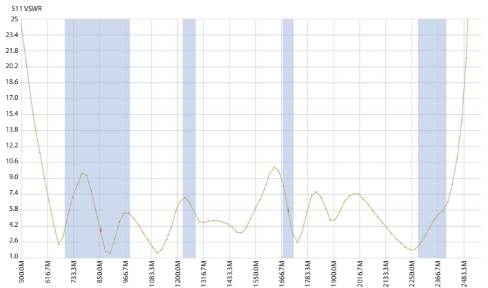
AN-E grafikon merenja antene
