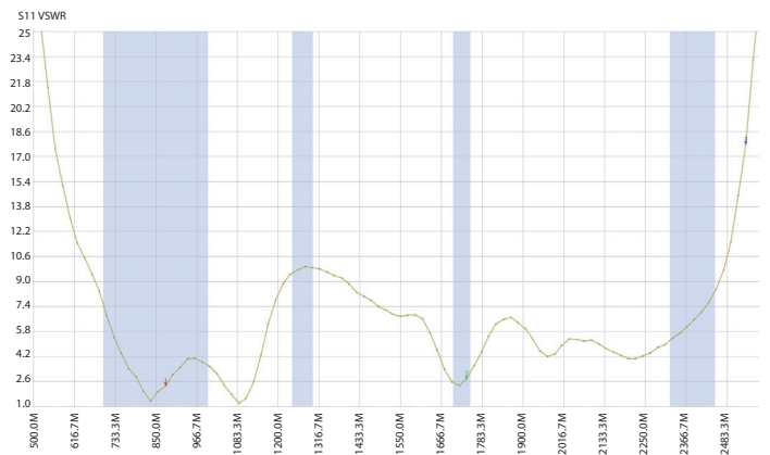
AN-E3 grafikon merenja antene
